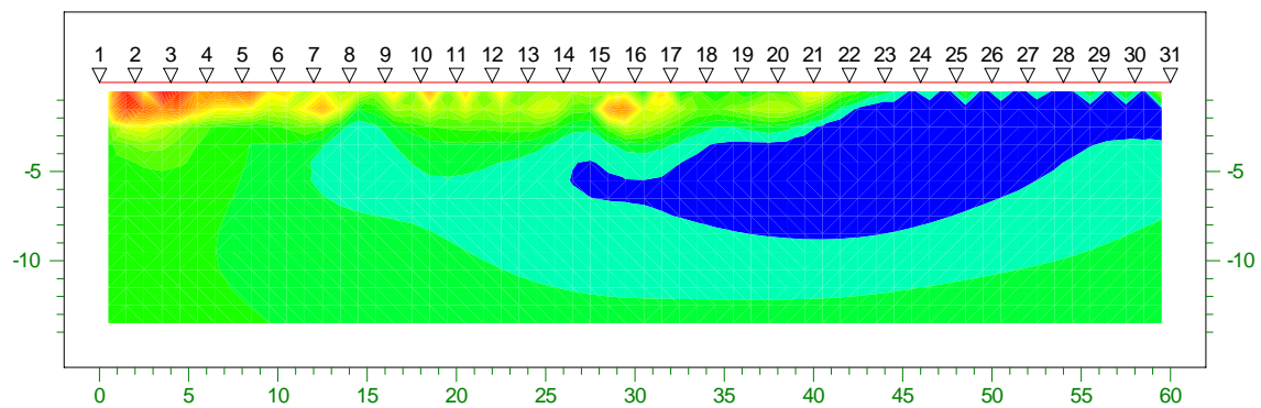
Sezione resistività modello inverso
