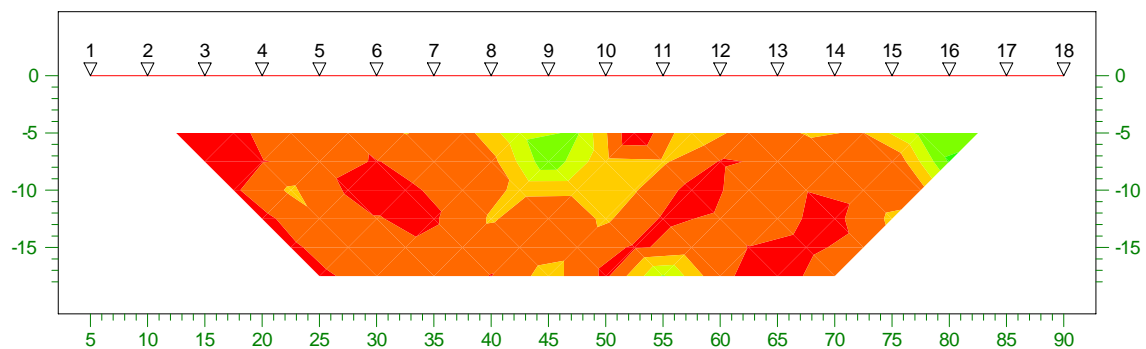
Pseudosezione resistività apparente
