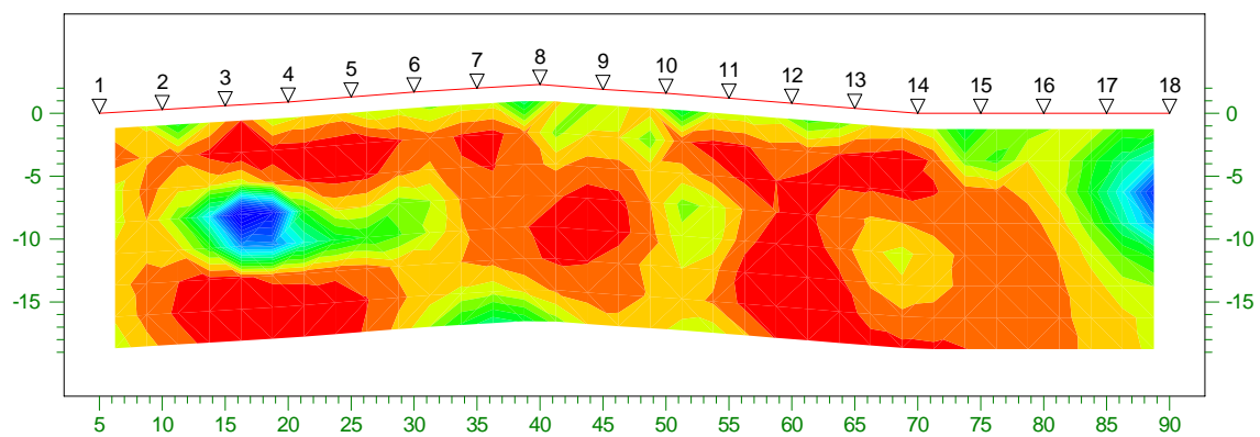
Sezione resistività modello inverso
