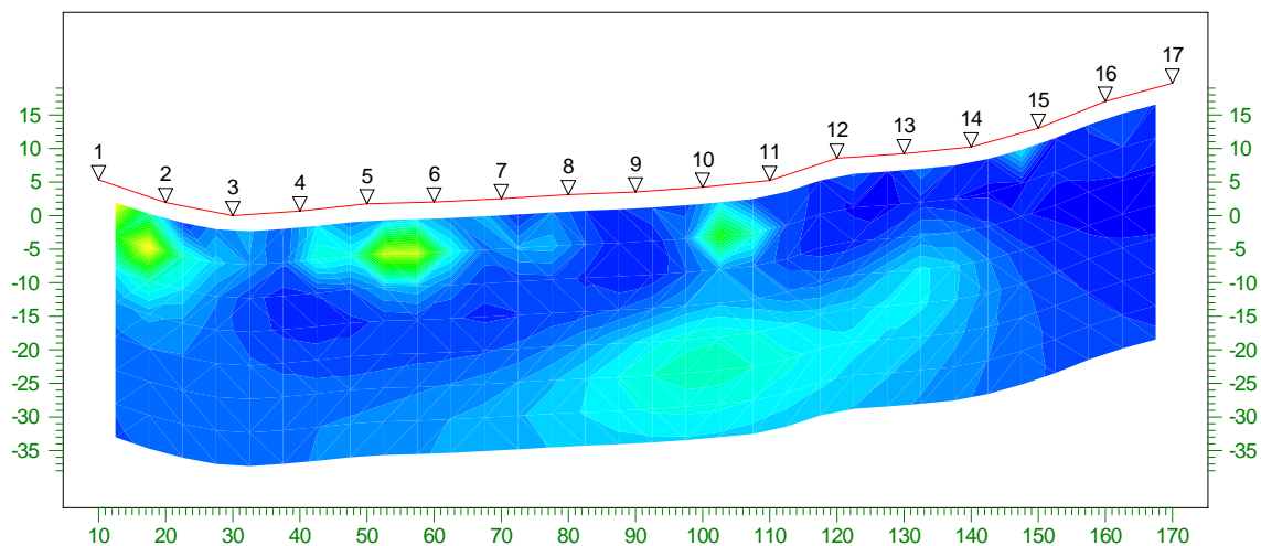
Sezione resistività modello inverso
