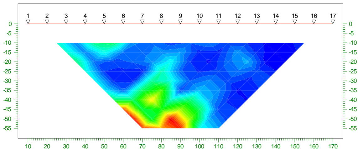
Pseudosezione resistività apparente
